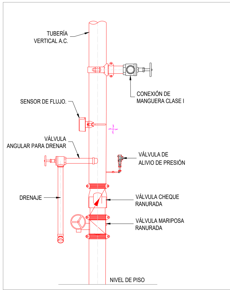
DETALLE PARA TUBERÍA VERTICAL PRIMER NIVEL SIN ESCALA
