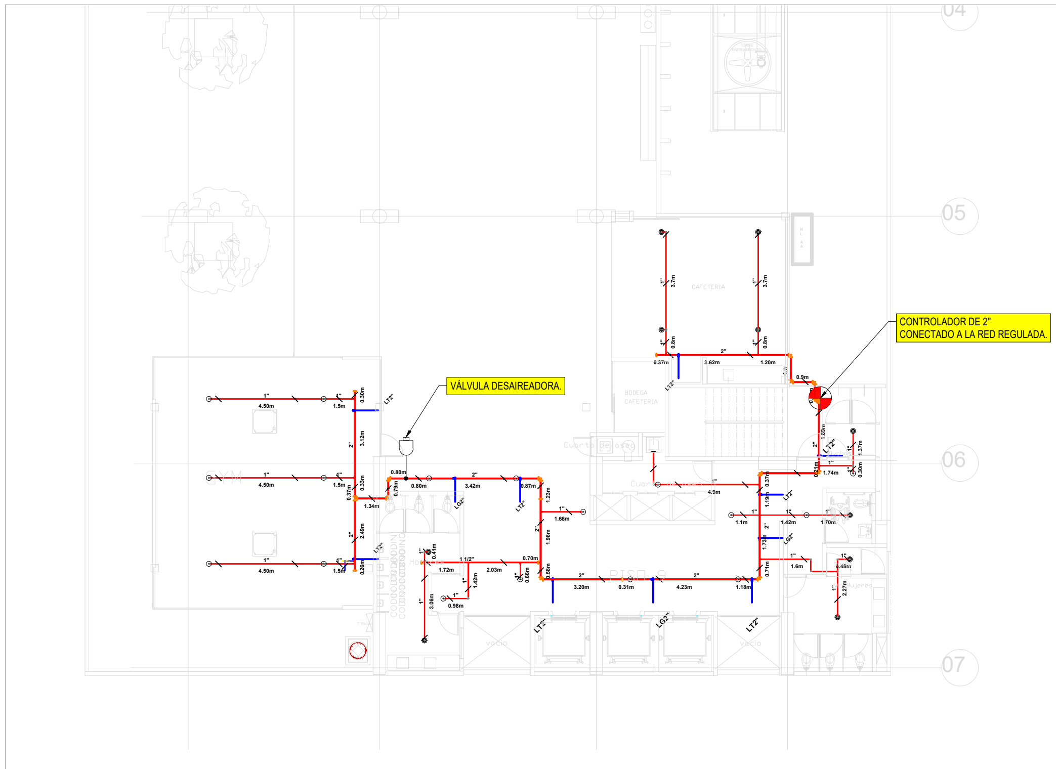
1 VISTA EN PLANTA EXTINCIÓN PISO 9 ESCALA 1:150
