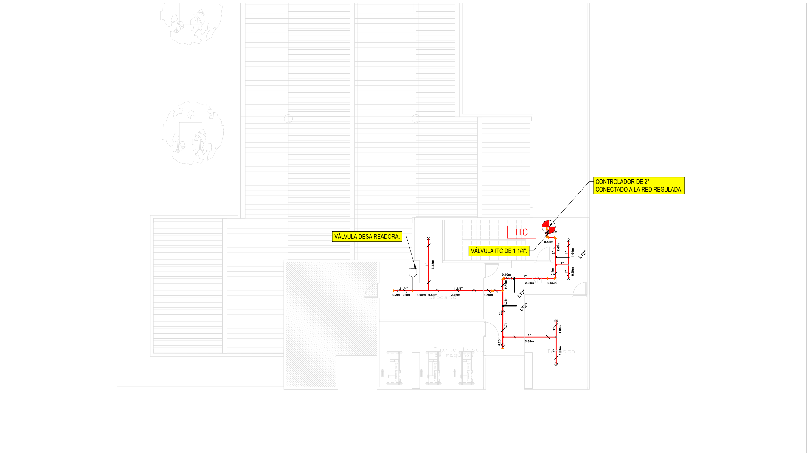
2 VISTA EN PLANTA EXTINCIÓN CUBIERTA ESCALA 1:150
